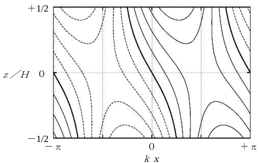
傾圧不安定波の流線関数の構造
