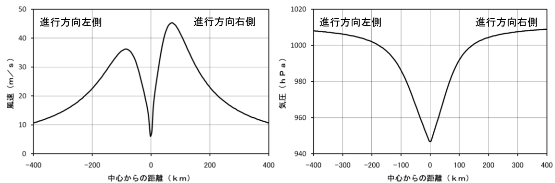
図11-3: 台風を中心のまわりの風速 (左) と気圧 (右) の分布の模式図
