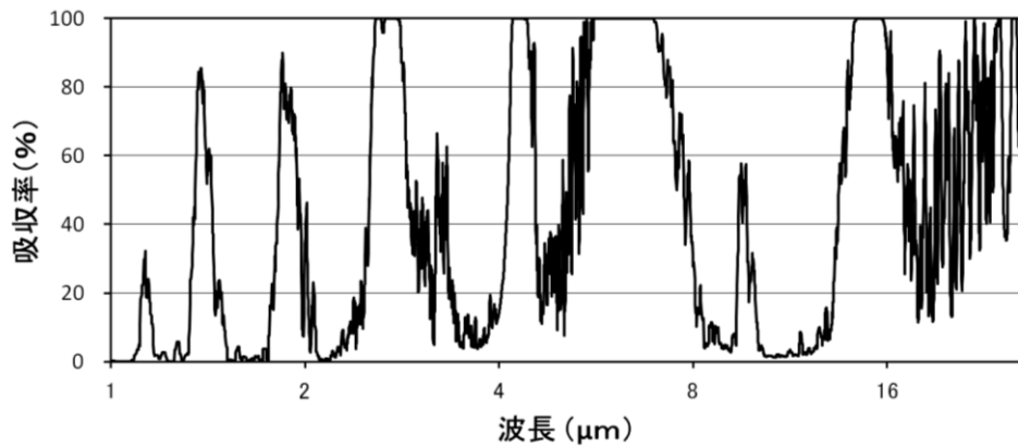
図 6-4: 放射に対する地球大気吸収率の計算例
