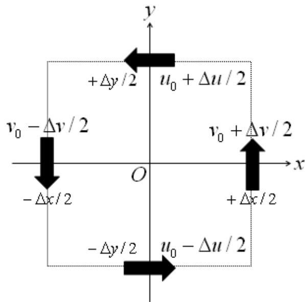
図 8-4: 渦度
